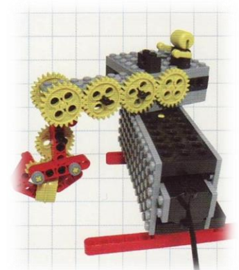
縦回転のギアを横の回転に変えるギアの組み方を学ぶ「ロボットアーム」
